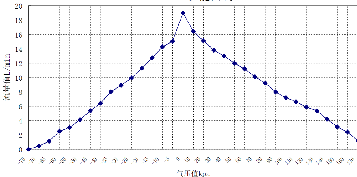
DA80RHDC12V性能曲线
