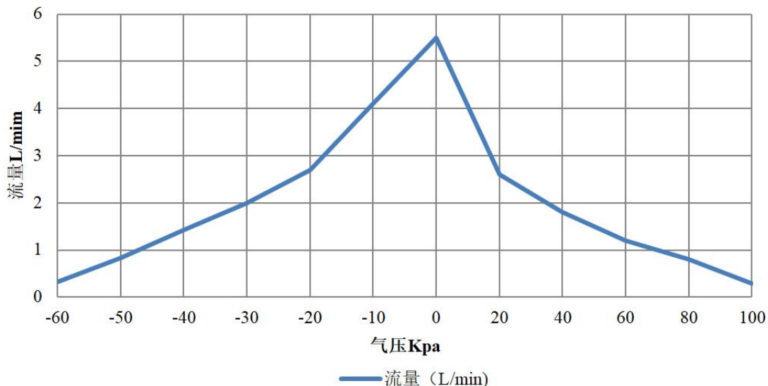
DA72AC4P性能曲线
