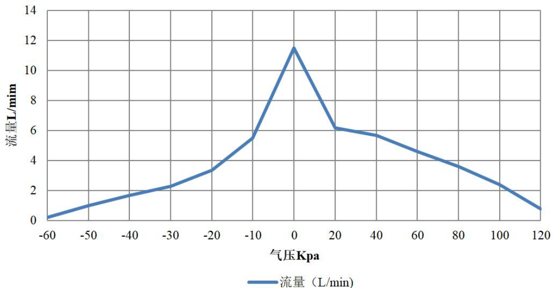
DA72AC220V2P性能曲线
