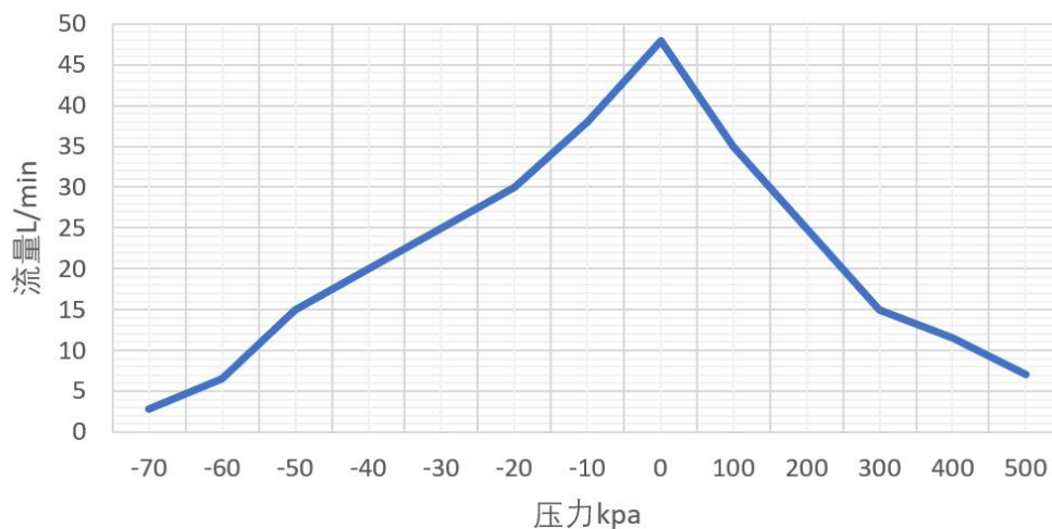
WA78流量
